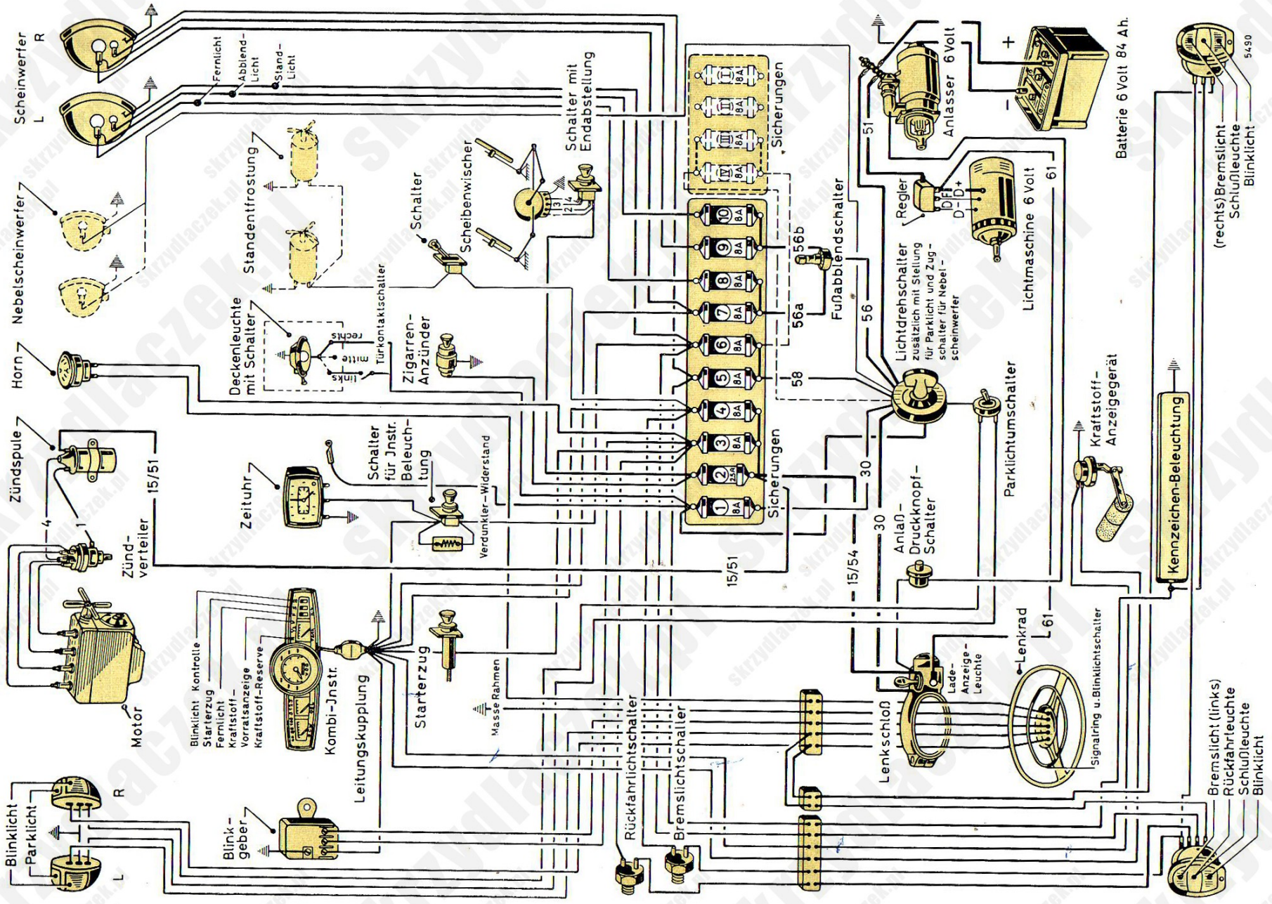
Schaltplan der elektrischen Einrichtungen
