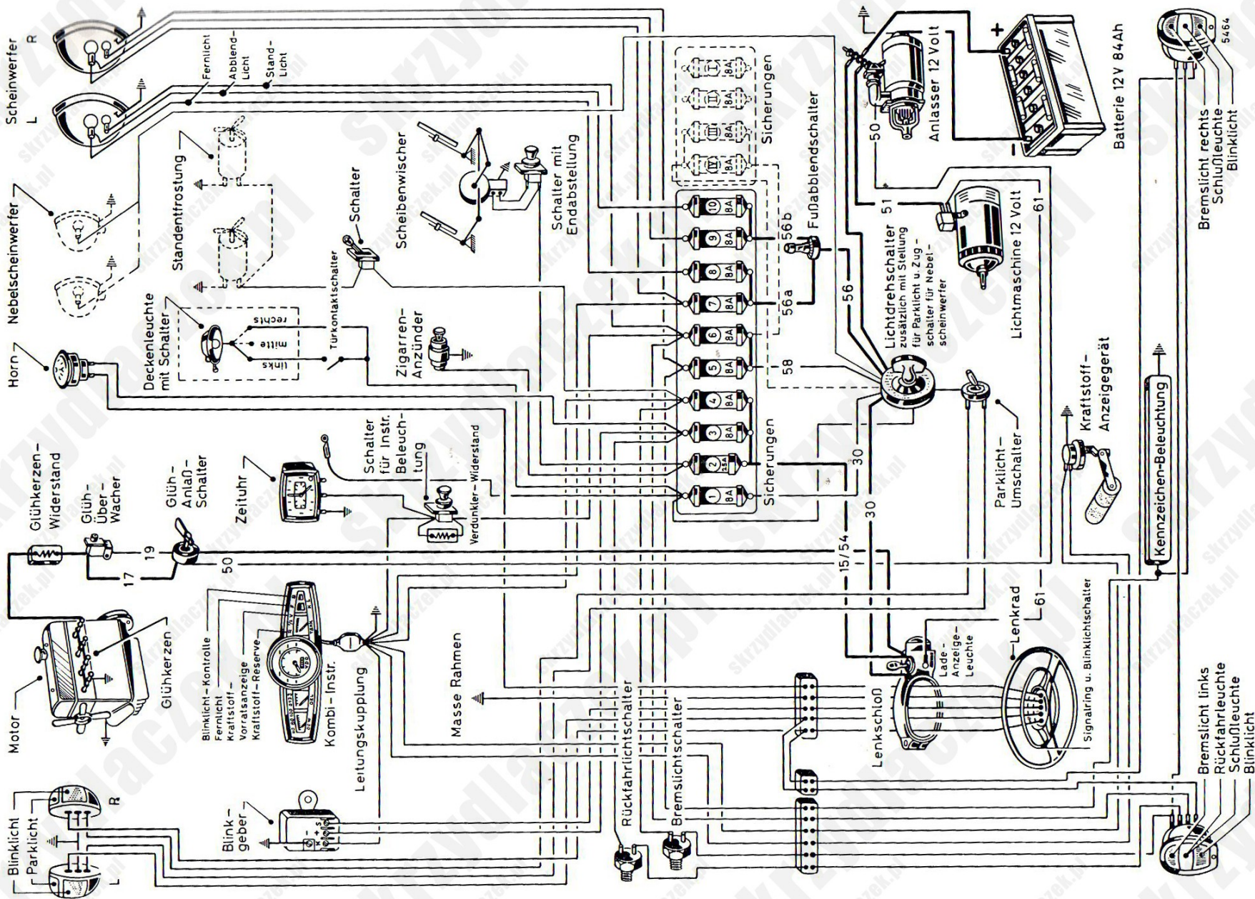
Schaltplan der elektrischen Einrichtungen
