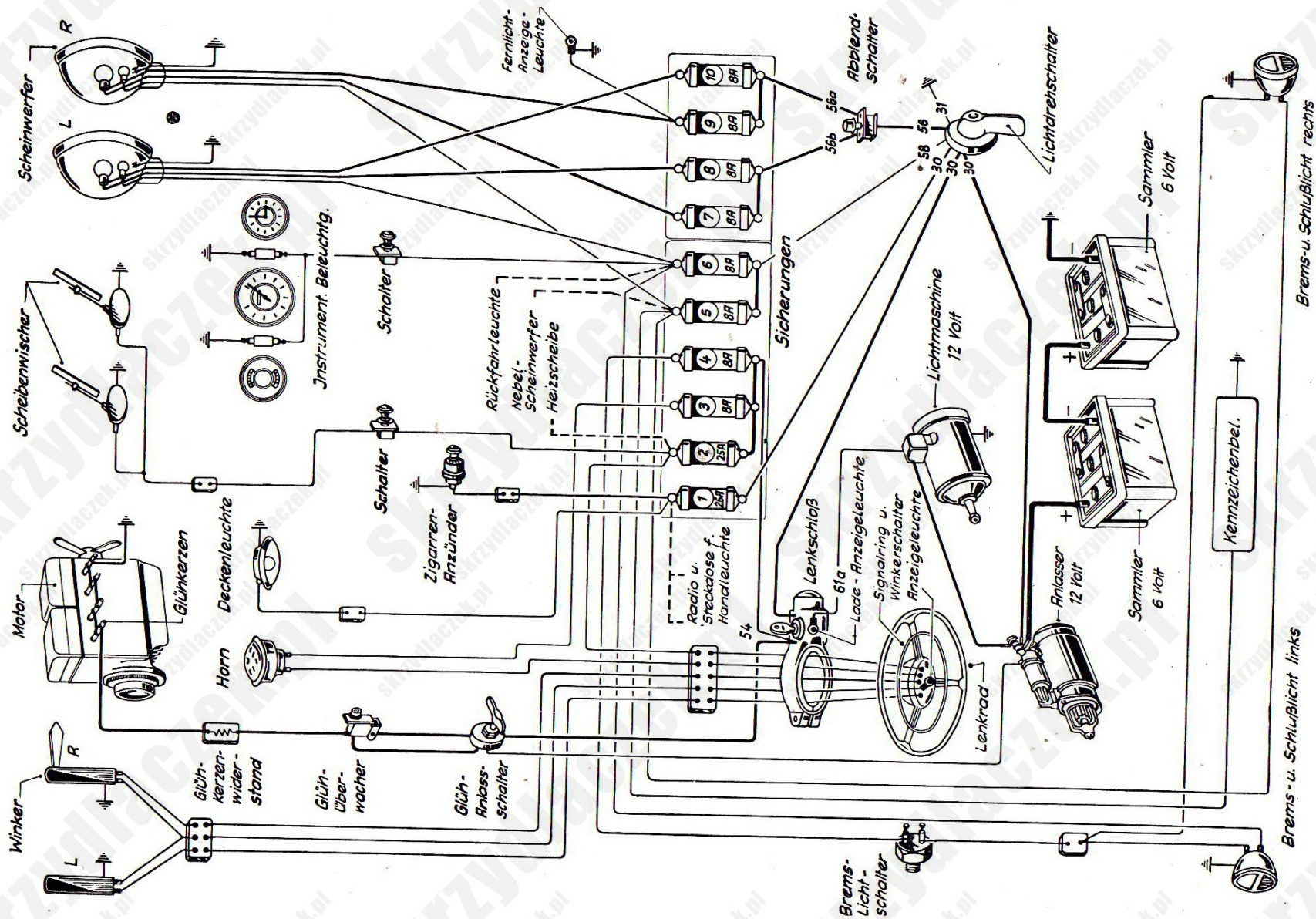
Schaltplan der elektrischen Einrichtung
